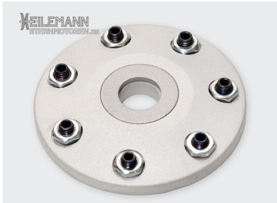
HS-Propellerdruckscheibe für 10mm-Welle Außendurchmesser 54mm
